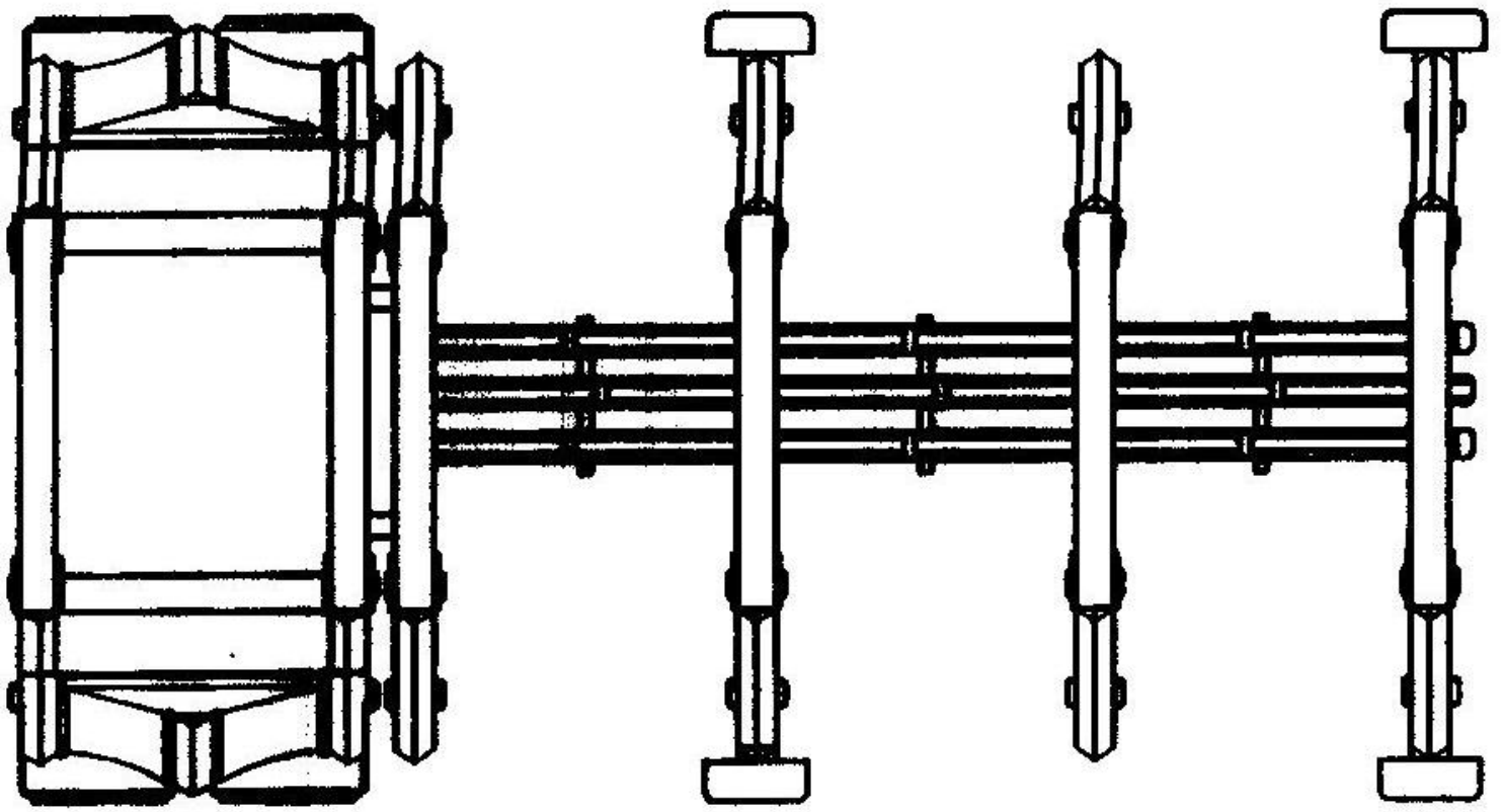
俯视图
