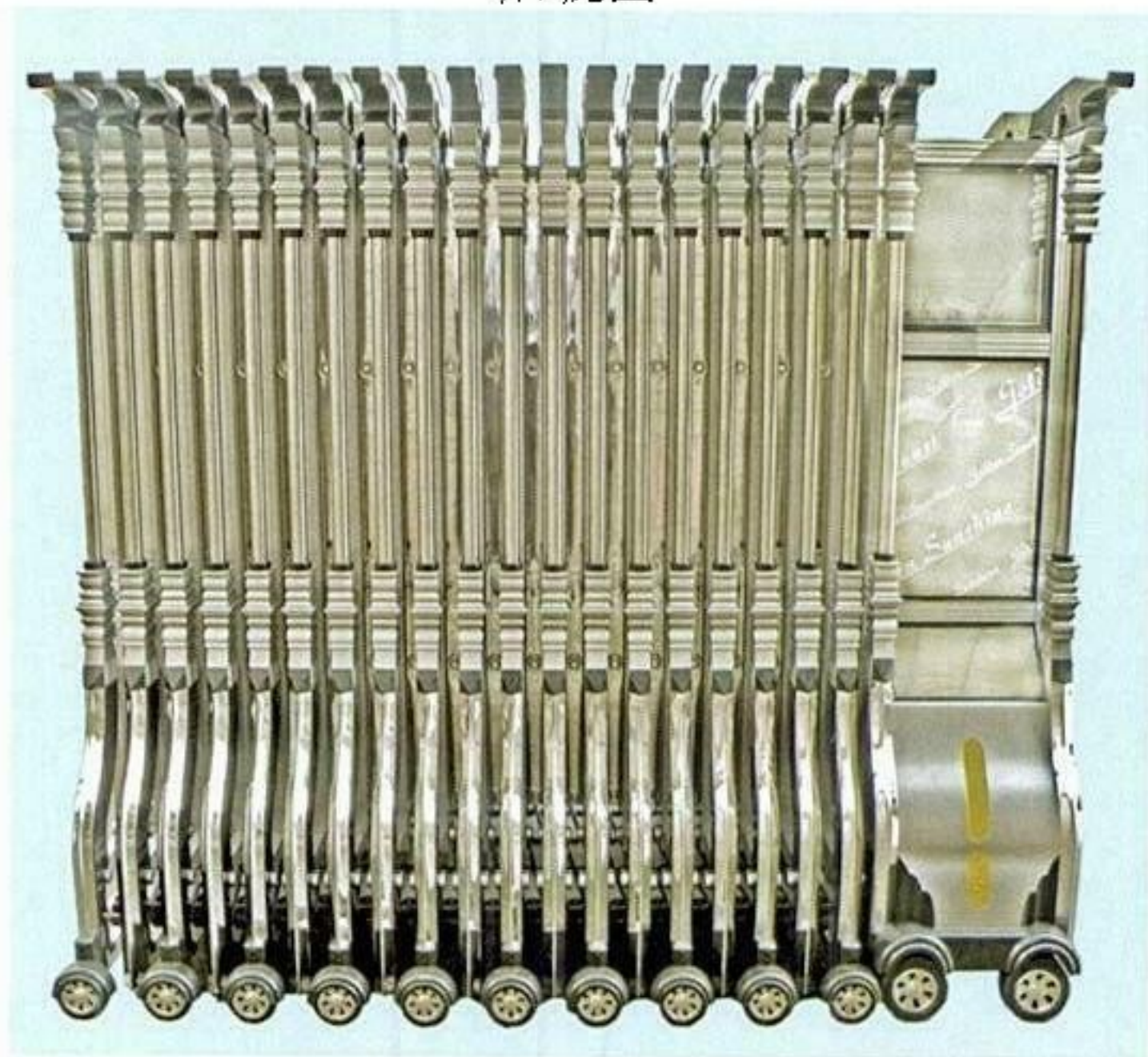
后视图
